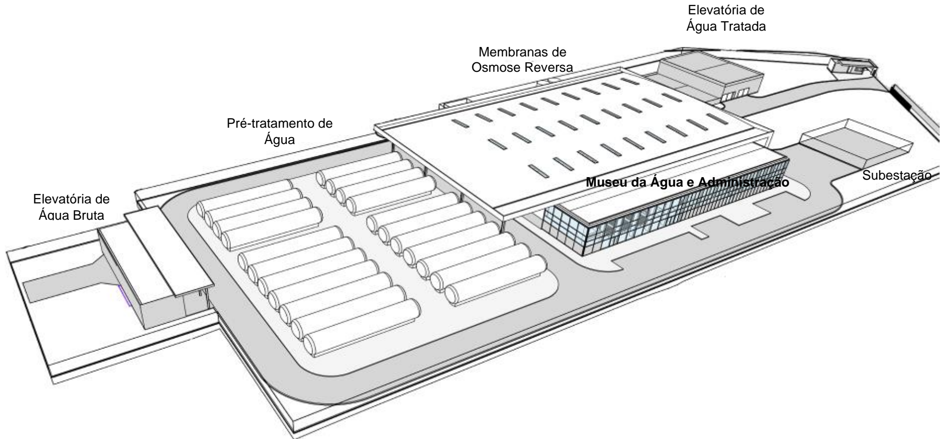
Figura 2. Perspectiva das principais unidades componentes da planta.
